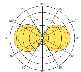
SLIM 2x...W
