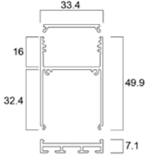
Perfil H 30 (33x50)
