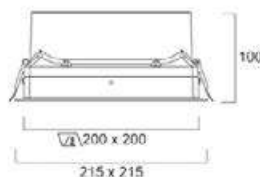
Solstice - Reflector plata - Bisel Blanco - Cuadrado
