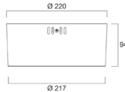
START Downlight 220 - Montaje superficie
