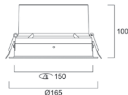
Solstice - Reflector negro - Bisel negro
