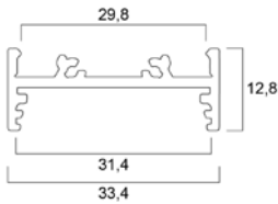
Perfil poco profundo para superficie ancha 30 (33x13)
