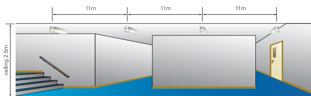
Colocar luminárias adicionais para atingir o mínimo de 1 lux
