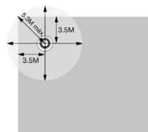
Distância máxima para evitar espaços sem cobertura
