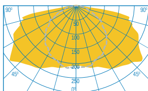
Posição fechada (II)
