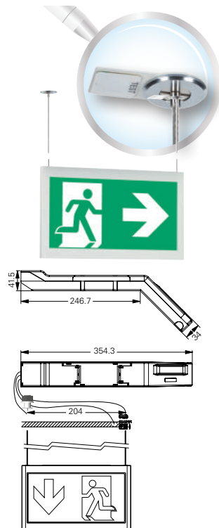
Detalhe do suporte para instalação suspensa com botão de teste e led de estado
