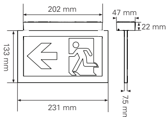
CrystalWay 30m - Montagem mural
