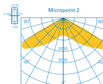
Área aberta (iluminação simétrica)
