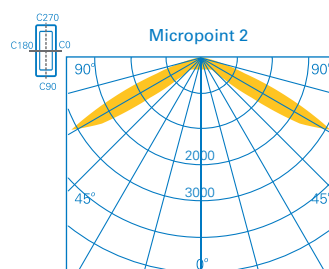
Caminho de evacuação (iluminação assimétrica)
