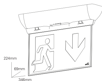
Montagem em suspensão
