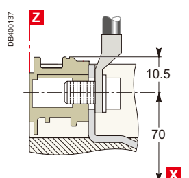
Cabos com terminais/barras
