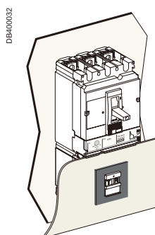
Moldura para módulo Vigi.
