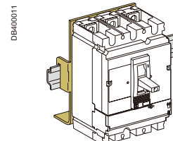
Montagem em calha DIN (com adaptador)
