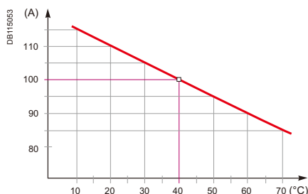
Curva de descarga de temperatura para CVS100.
