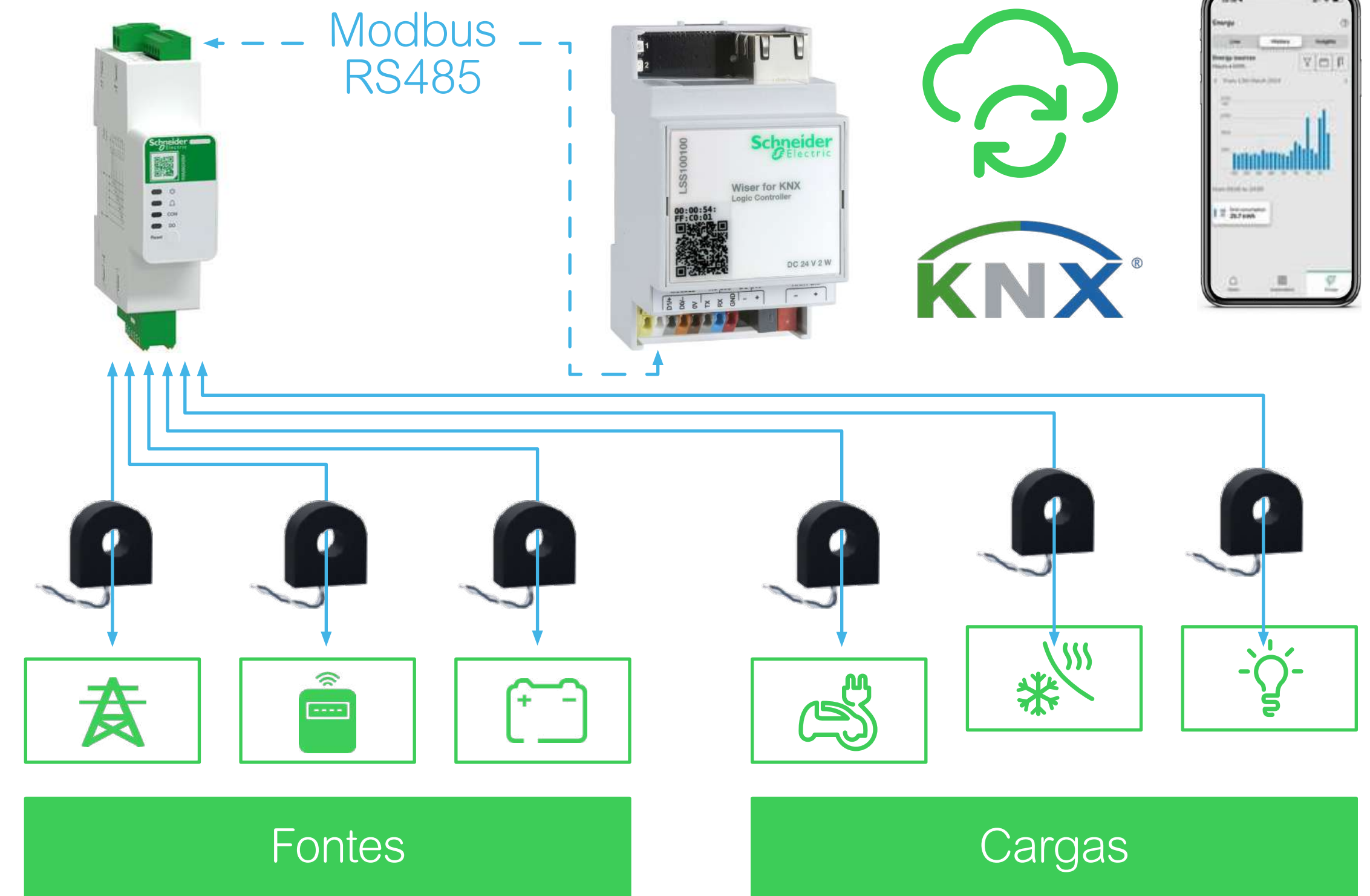
Contador de energia Resi9 com fios
